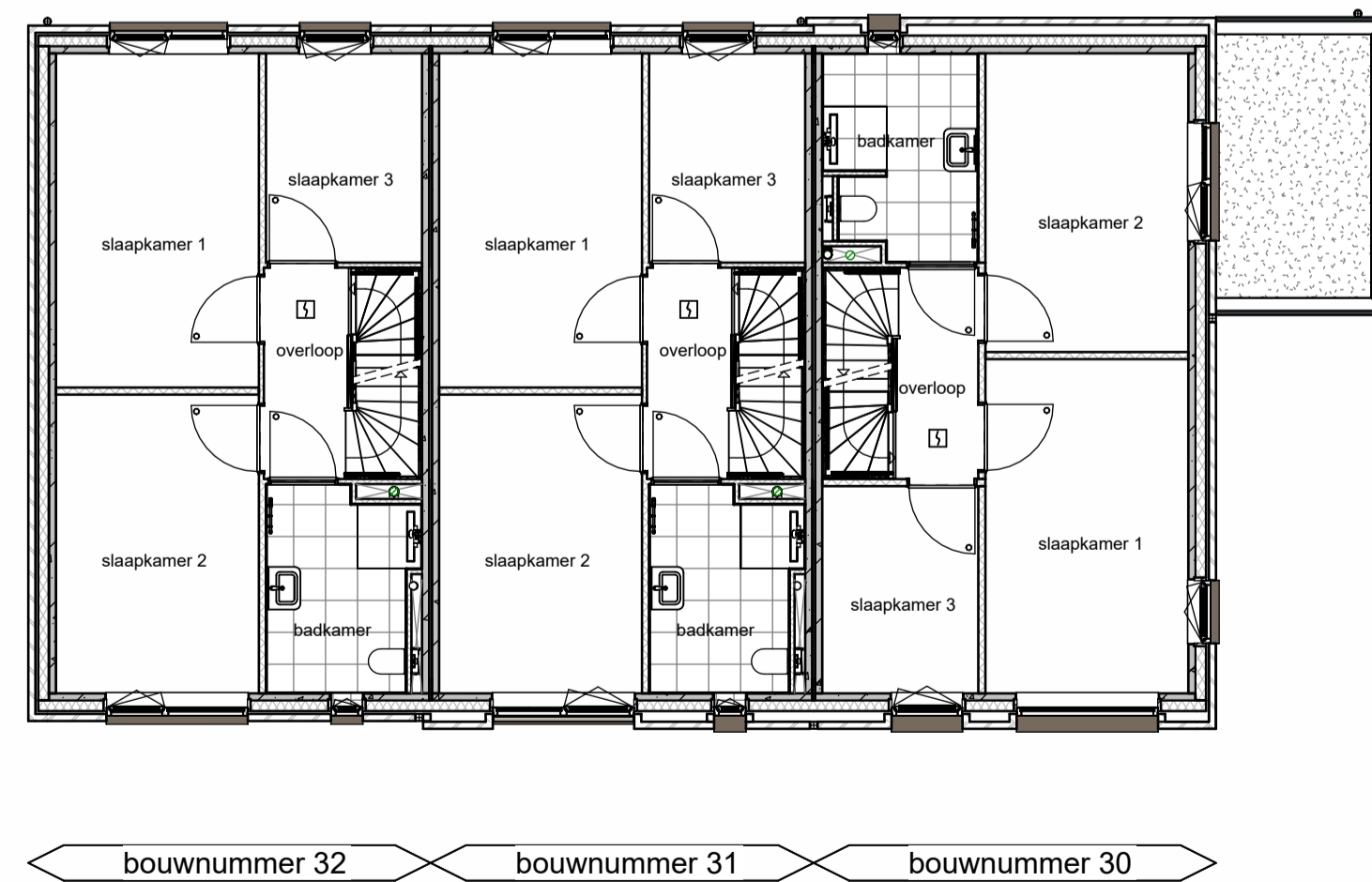
1e verdieping
