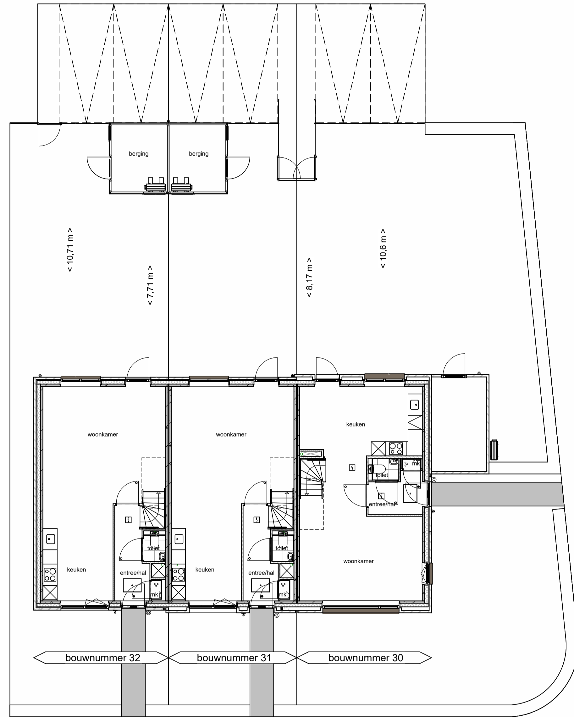
Begane grond
