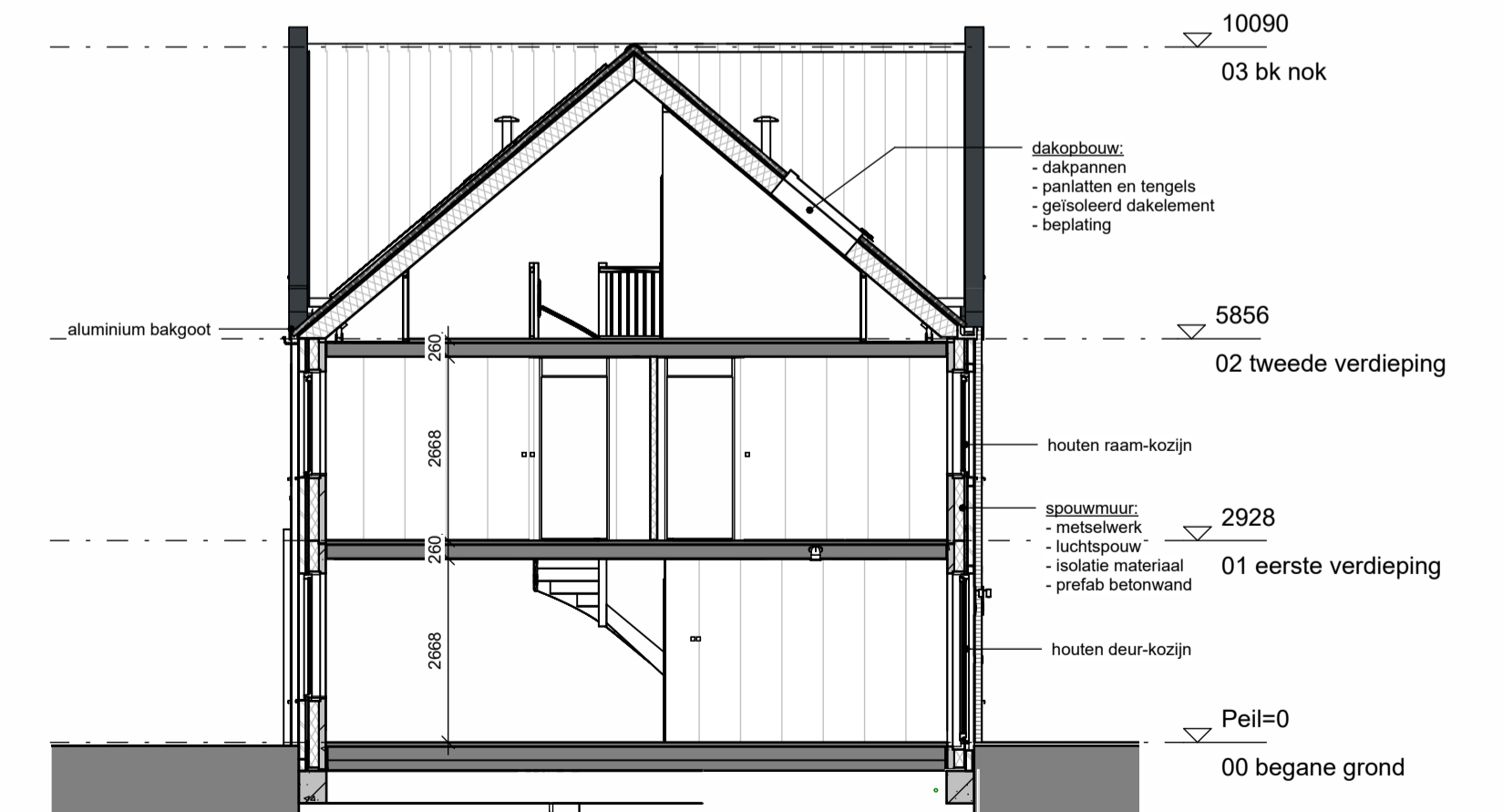
Doorsnede Bnr 32
