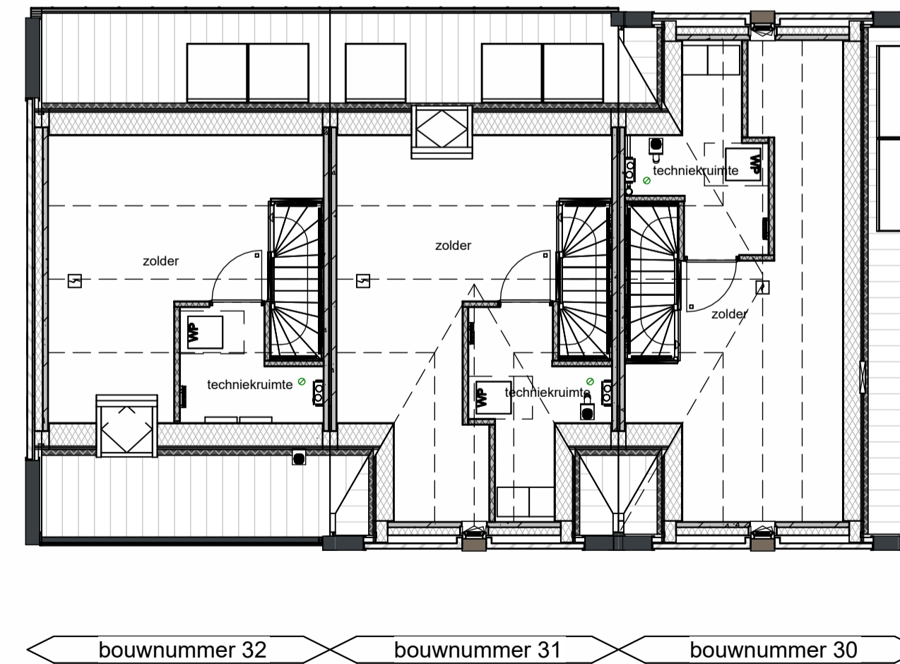
2e verdieping
