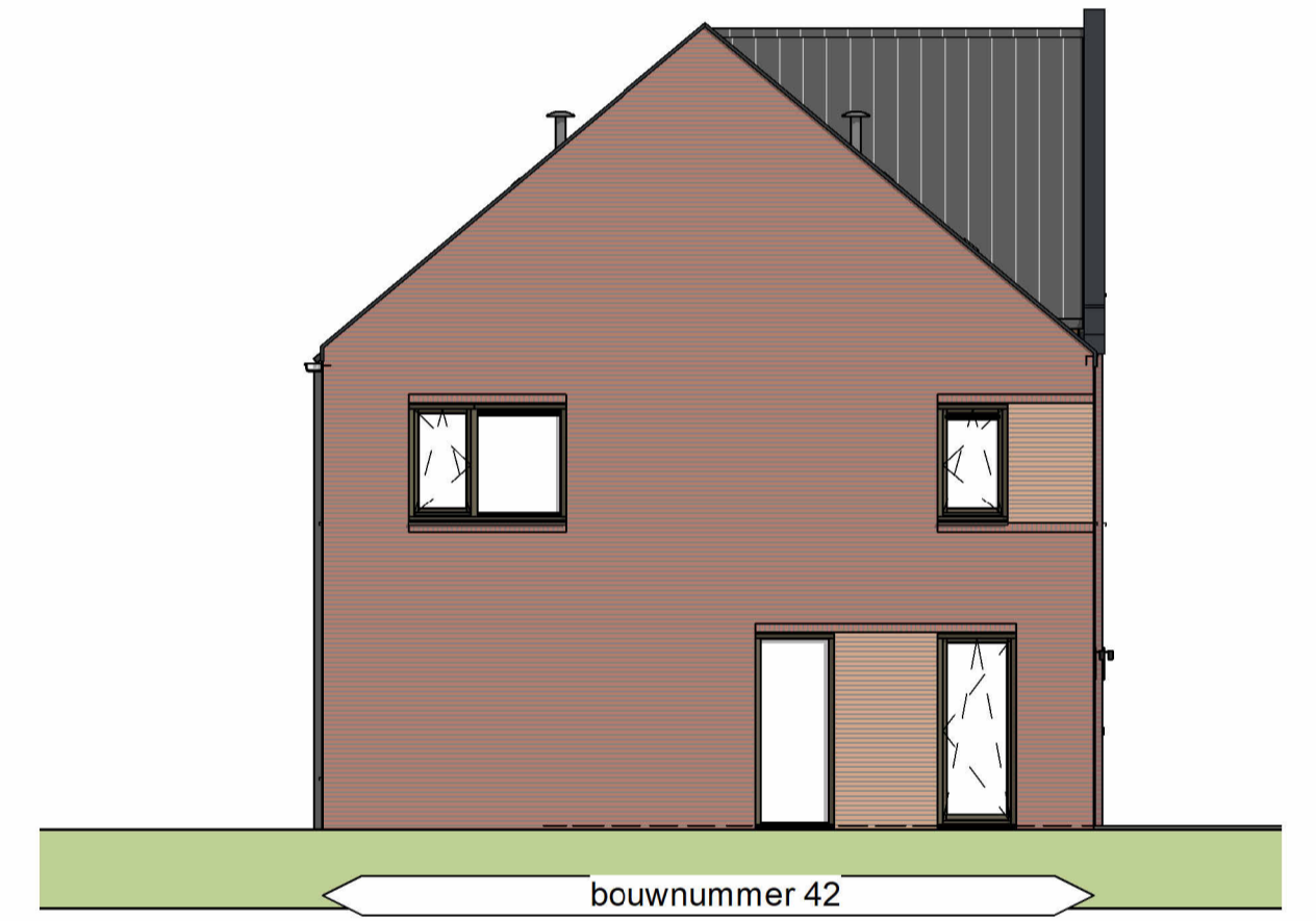
Linker zijgevel - Blok 38.42 1op100
