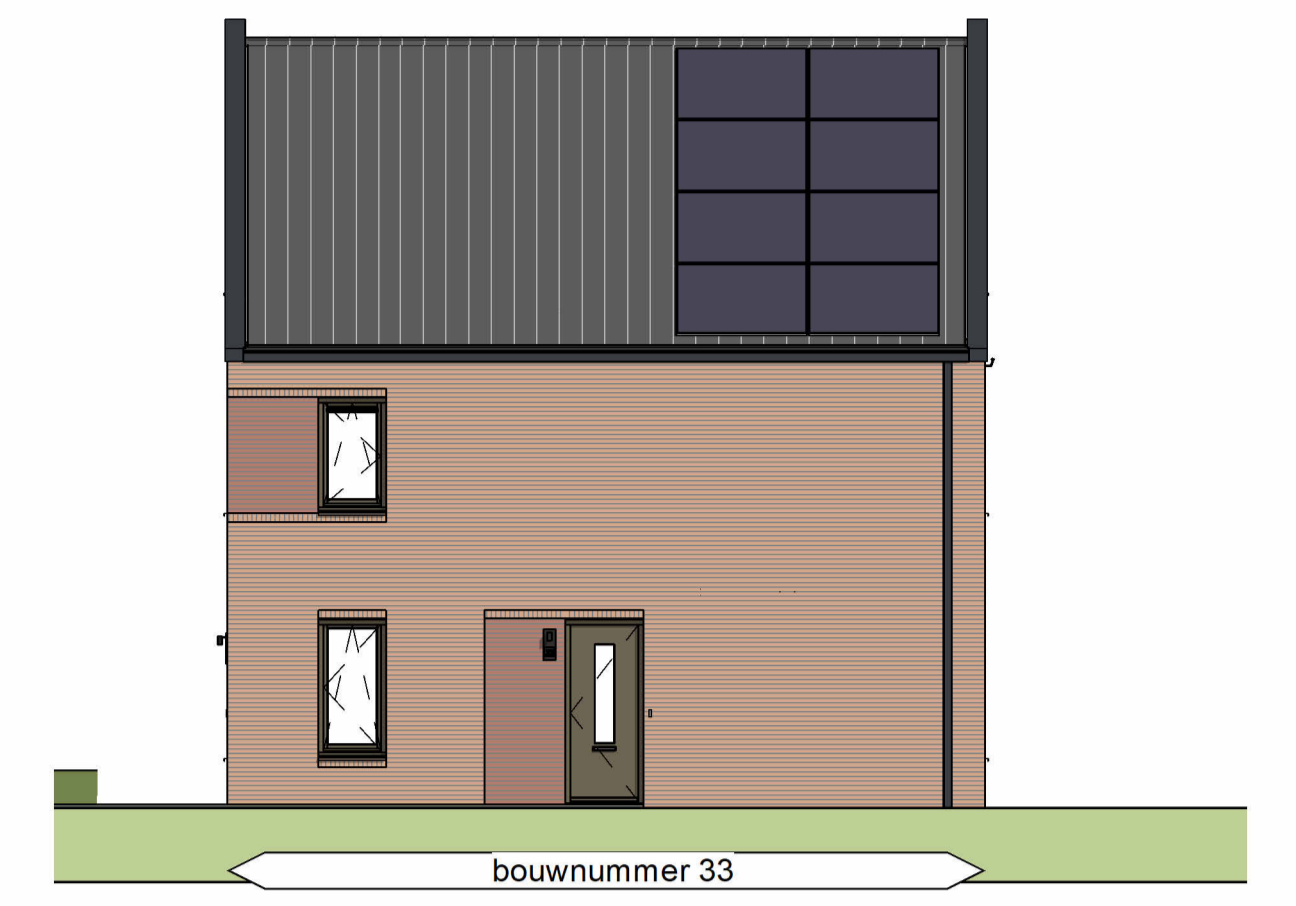
Rechter zijgevel
