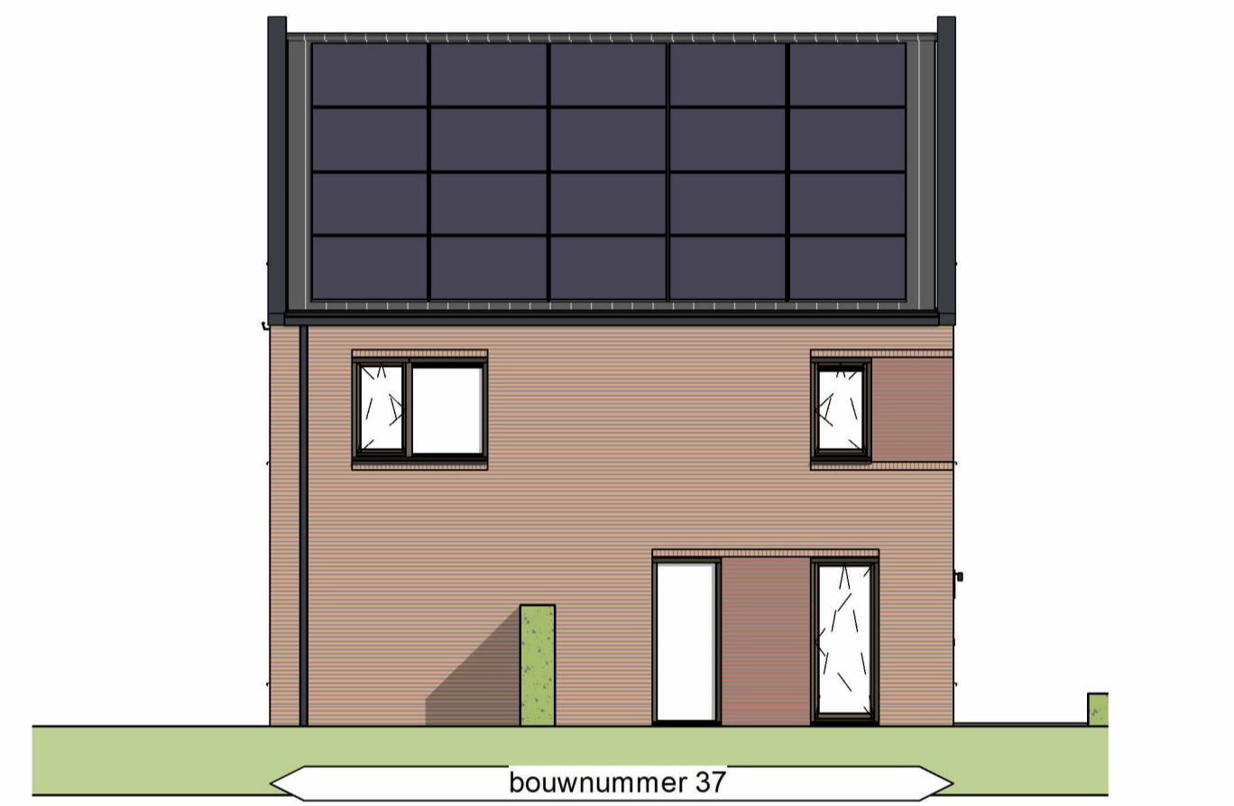
Linker zijgevel
