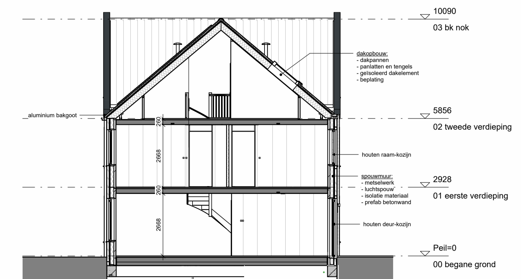
Doorsnede Bnr 33.37
