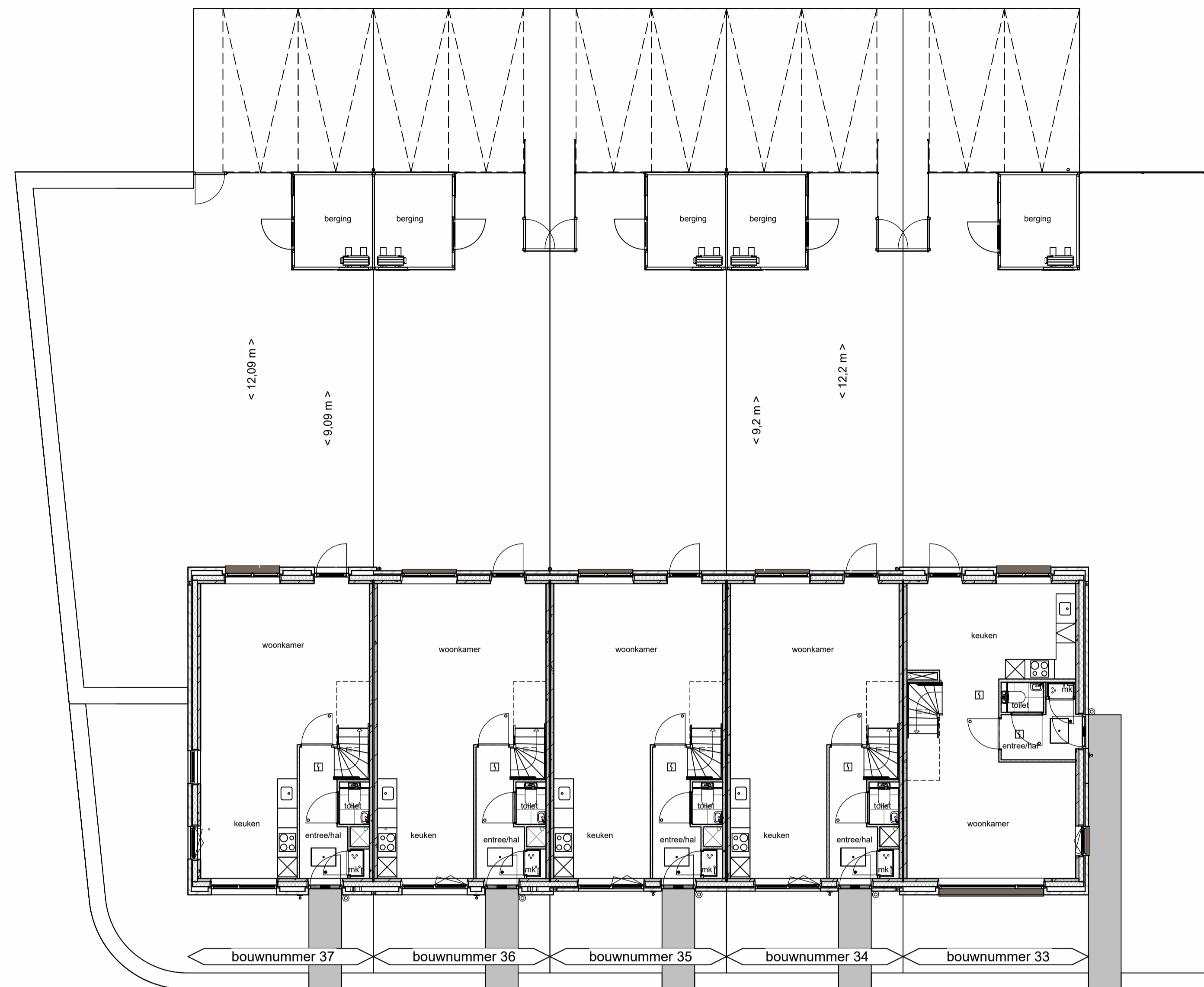
Begane grond
